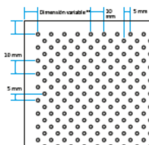
Perforación \varnothing 2,5 mm Área perforada ~ 10%
