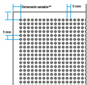
Perforación \varnothing 2,5 mm Área perforada ~ 20%
