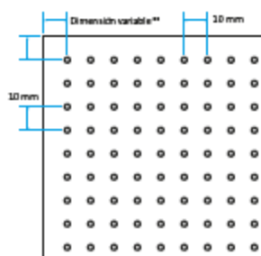
Perforación \varnothing 2,5 mm Área perforada ~ 5%
