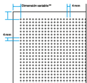
Perforación \varnothing 1,5 mm Área perforada ~ 11%
