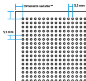
Perforación \varnothing 2,5 mm Área perforada ~ 16%
