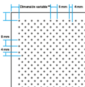
Perforación \varnothing 1,5 mm Área perforada ~ 11%
