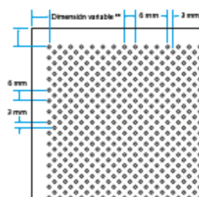
Perforación \varnothing 2 mm Área perforada ~ 18%
