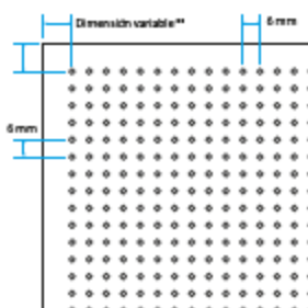
Perforación \varnothing 2 mm Área perforada ~ 9%
