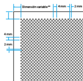
Perforación \varnothing 1,5 mm Área perforada ~ 22%
