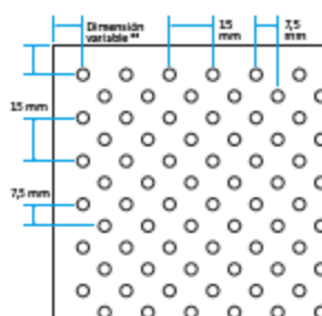
Perforación \varnothing 4 mm Área perforada ~ 11%
